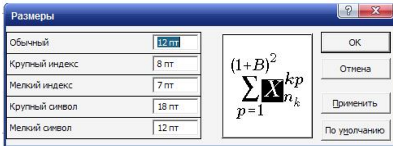
Рисунок 2 – Розміри формул
